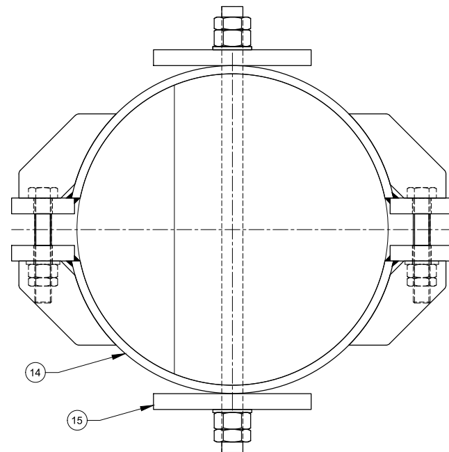
SECTION A-A Scale 1:5
